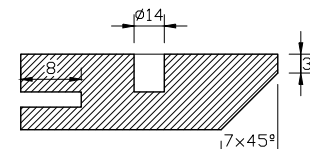
Cotas pequeñas Cotas dentro de trama Ángulo de 45°
