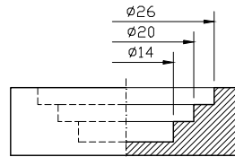
Diámetros en semicorte
